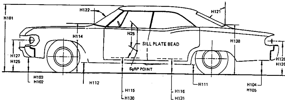
φFIG. 20—EXTERIOR DIMENSIONS, HEIGHT
