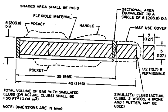
φFIG. 32—GOLF BAG
