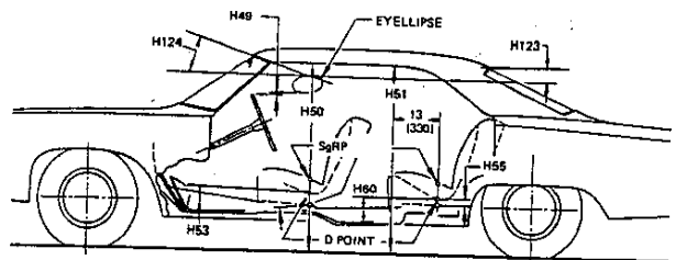
φFIG. 4—INTERIOR DIMENSIONS, HEIGHT
