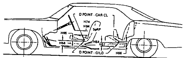
φFIG. 6—INTERIOR DIMENSIONS, HEIGHT
