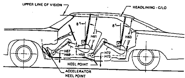
φFIG. 5—INTERIOR DIMENSIONS, HEIGHT
