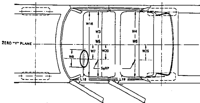
φFIG. 14—INTERIOR DIMENSIONS, WIDTH
