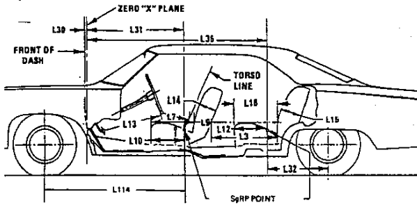
φFIG. 11—INTERIOR DIMENSIONS, LENGTH
