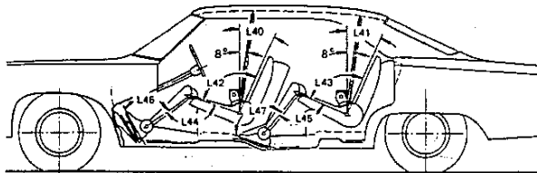
φFIG. 13—INTERIOR DIMENSIONS, LENGTH
